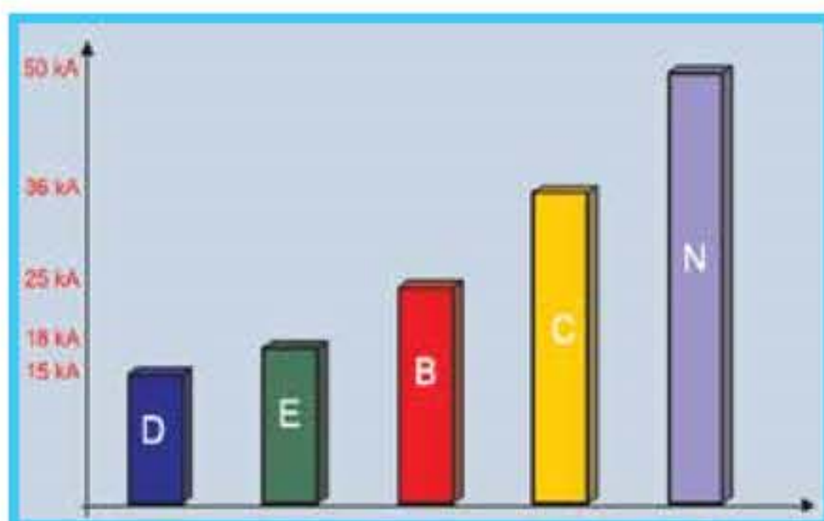
BZM2.. 125-250AT (25,36 kA)
